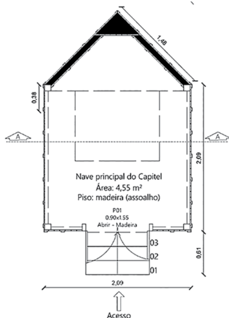
Figura 04 – Planta Baixa do Capitel Marini
