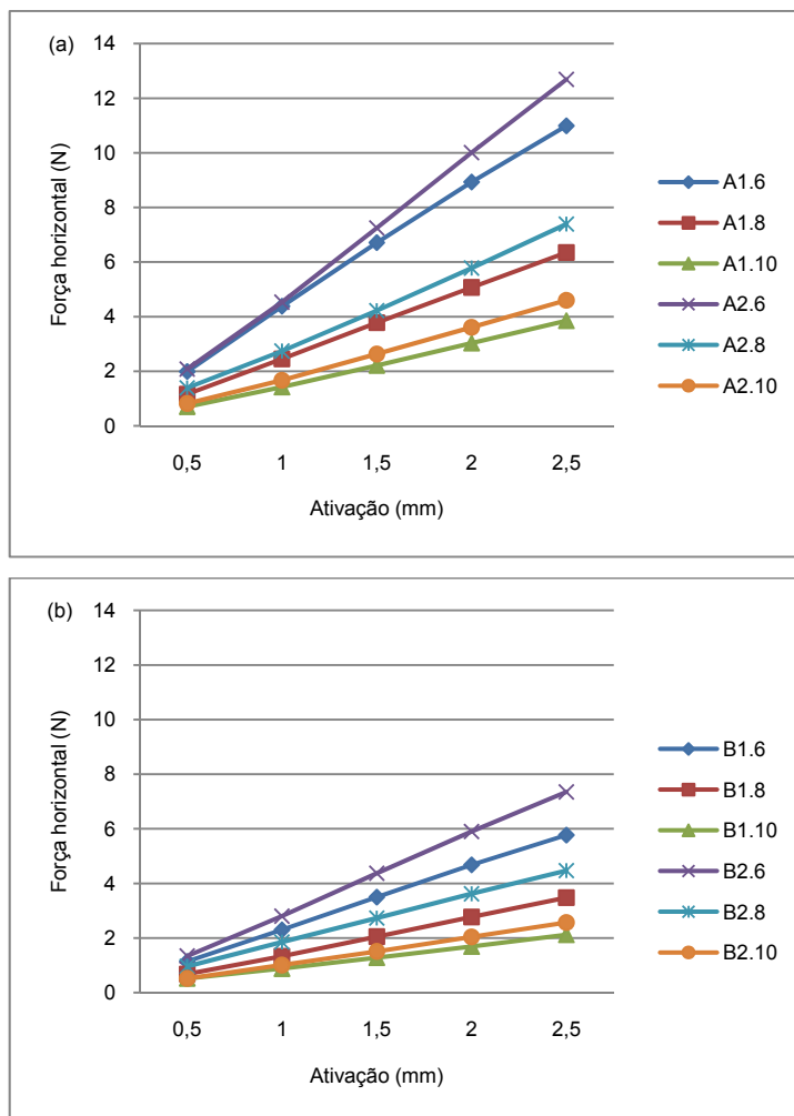
Figura 3 – Tendência da força média (N) das (a) alças de retração de aço inoxidável e das (b) alças de retração de beta-titânio (TMA).
