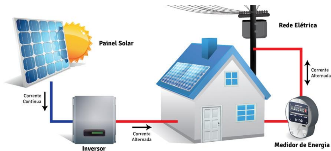
Figura 1 – Esquema de instalação de um sistema fotovoltaico em uma residência
