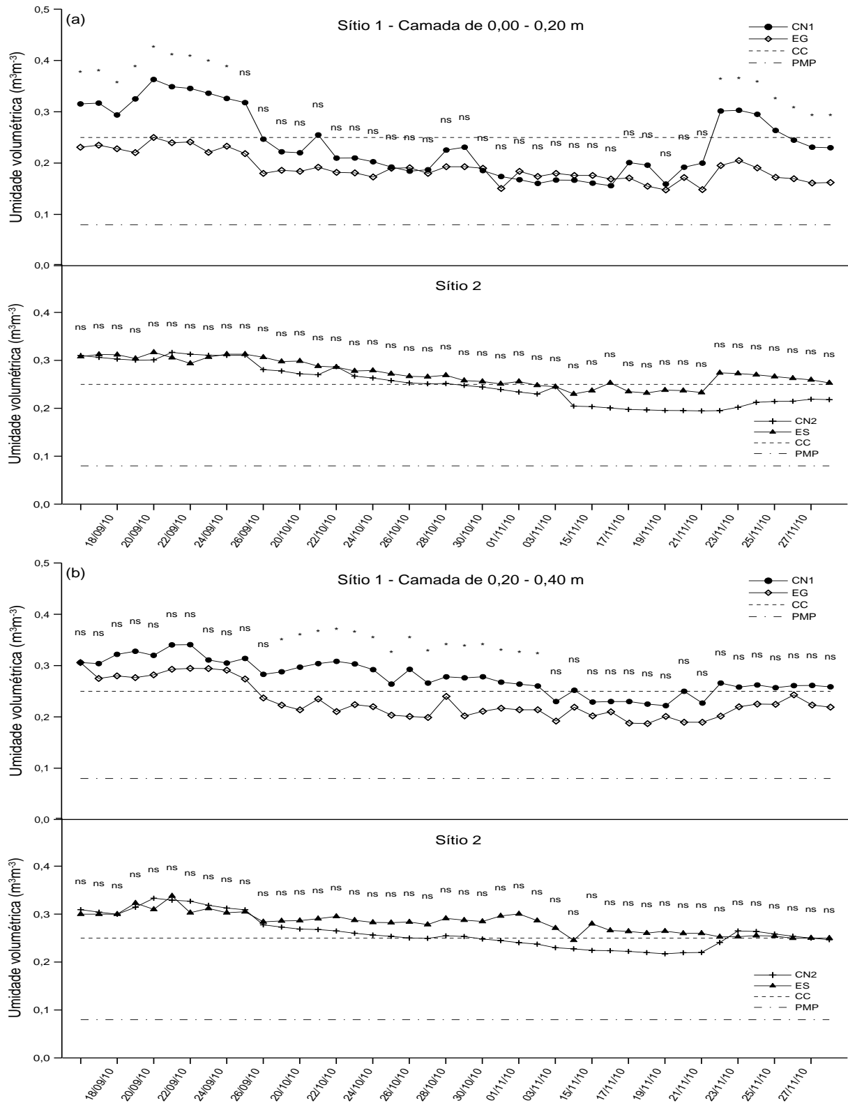
Figura 23 - Umidade volumétrica na Primavera nas camadas de (a) 0,00 a 0,20 m e (b) 0,20 a 0,40 m para os diferentes usos do solo.
