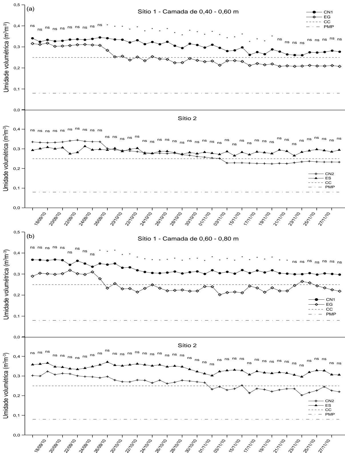
Figura 24 - Umidade volumétrica na Primavera nas camadas de (a) 0,40 a 0,60 m e (b) 0,60 a 0,80 m para os diferentes usos do solo.
