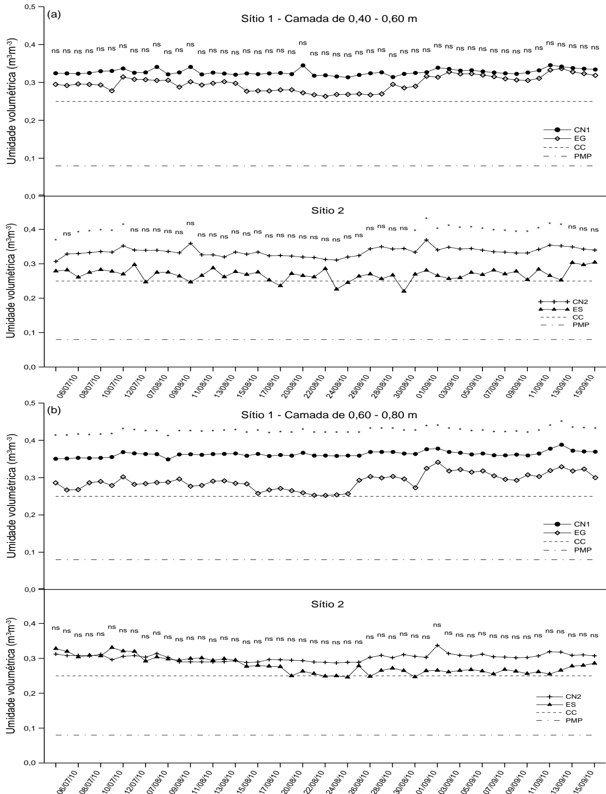
Figura 21 - Umidade volumétrica no Inverno nas camadas de (a) 0,40 a 0,60 m e (b) 0,60 a 0,80 m para os diferentes usos do solo.
