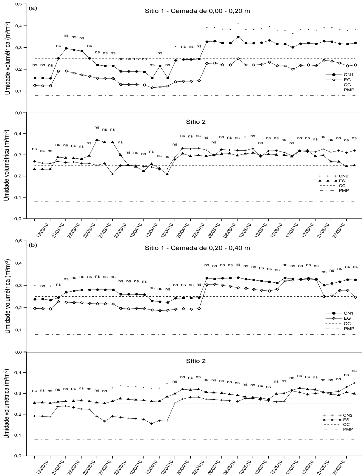
Figura 17 - Umidade volumétrica no Outono nas camadas de (a) 0,00 a 0,20 m e (b) 0,20 a 0,40 m para os diferentes usos do solo.
