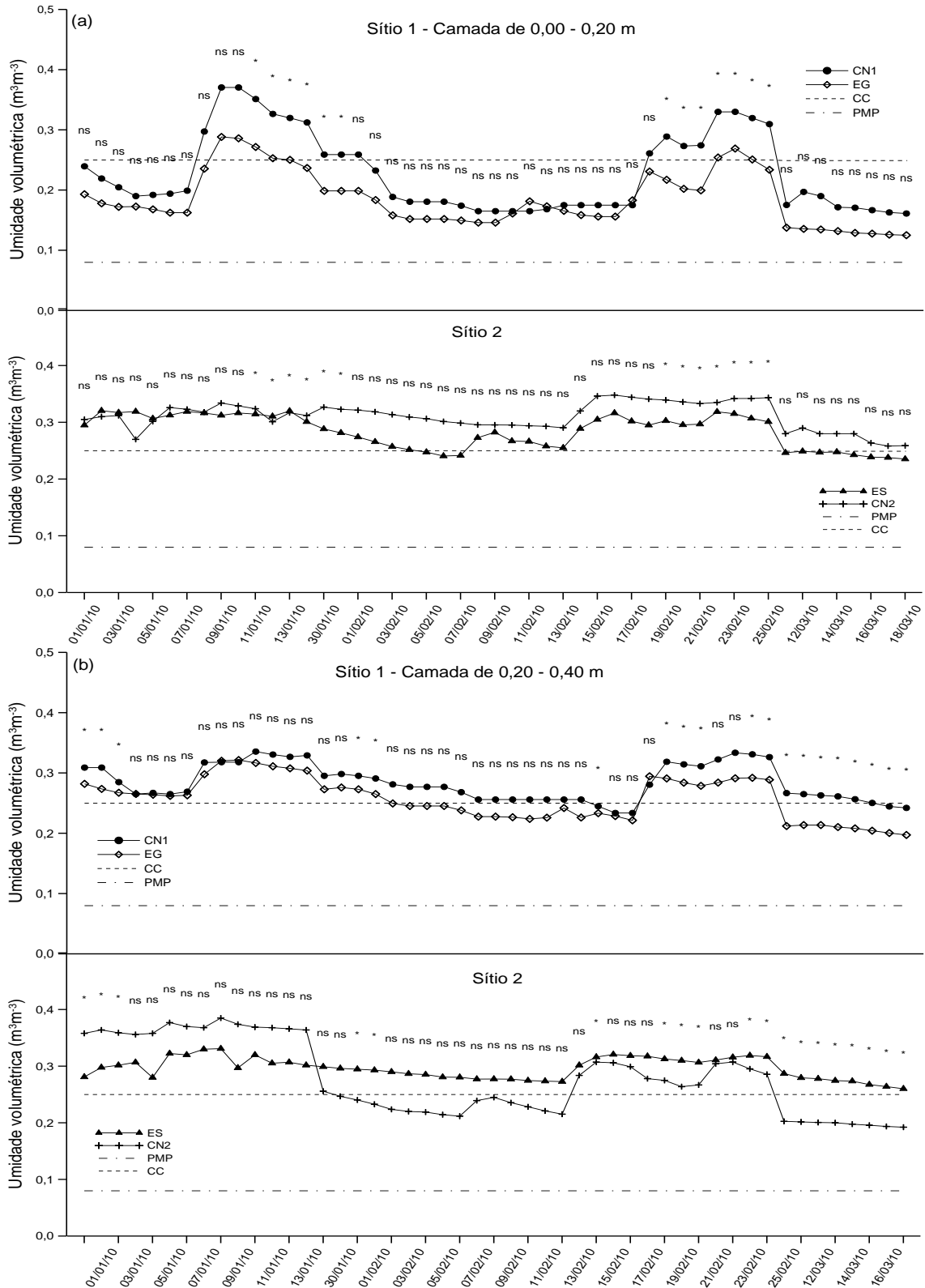
Figura 14 - Umidade volumétrica no Verão nas camadas de (a) 0,00 – 0,20 m e (b) 0,20 – 0,40 m para os diferentes usos do solo.
