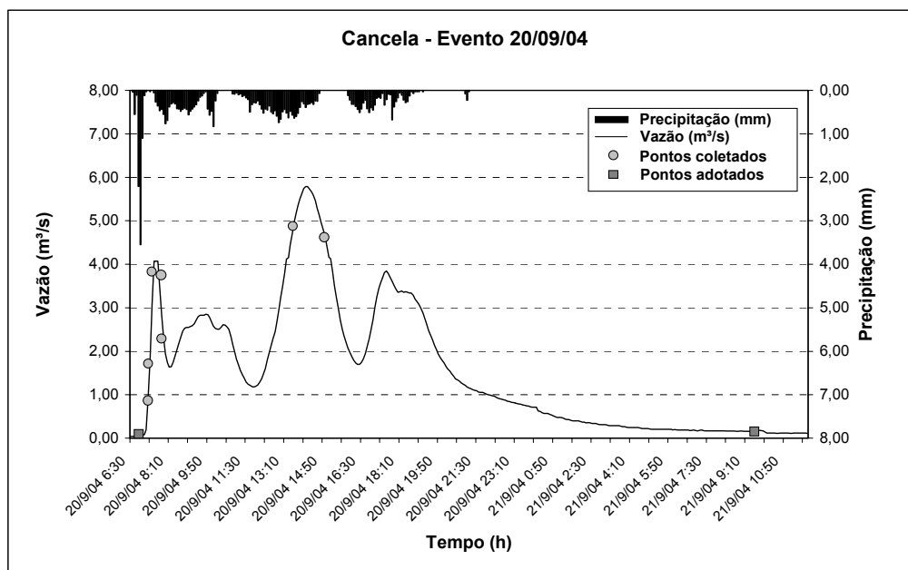
FIGURA 76 – Hidrograma do Evento 20/09/04 – Bacia Hidrográfica Cancela
