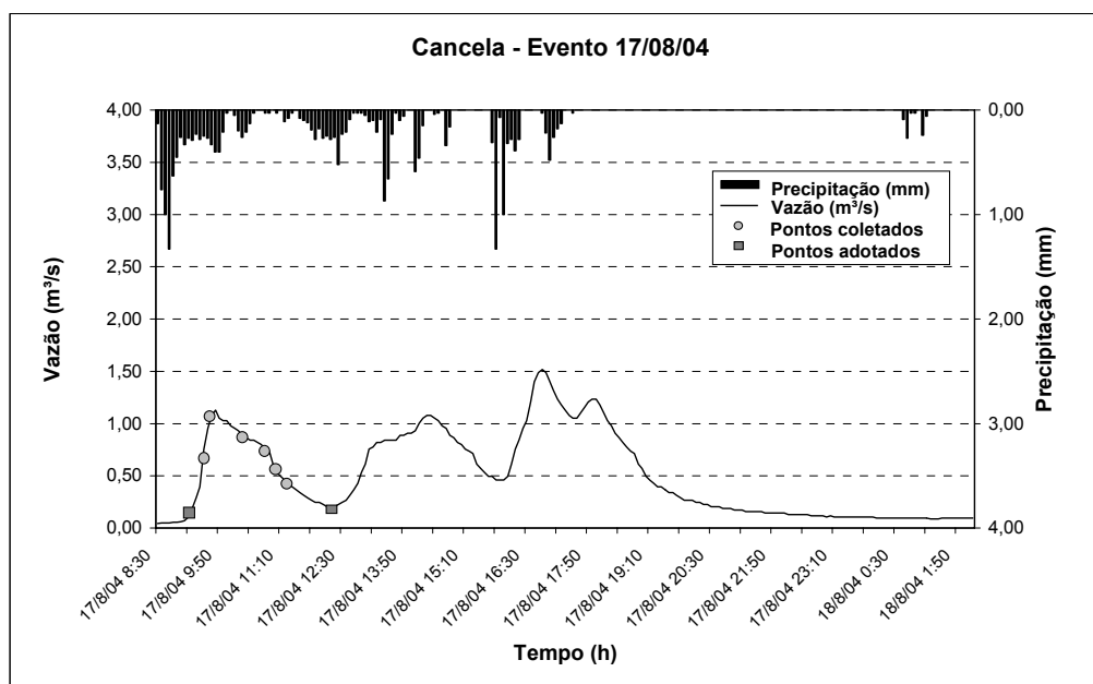
FIGURA 74 – Hidrograma do Evento 17/08/04 – Bacia Hidrográfica Cancela
