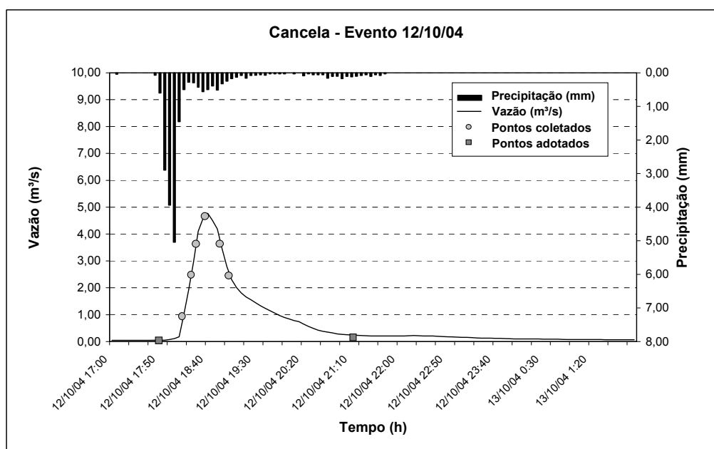
FIGURA 77 – Hidrograma do Evento 12/10/04 – Bacia Hidrográfica Cancela
