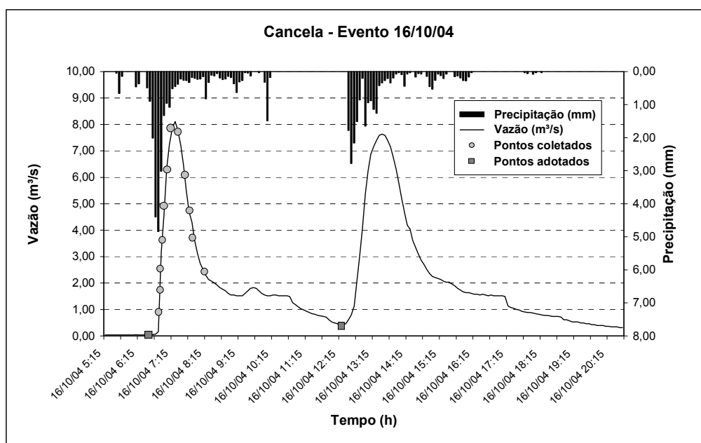
FIGURA 78 – Hidrograma do Evento 16/10/04 – Bacia Hidrográfica Cancela
