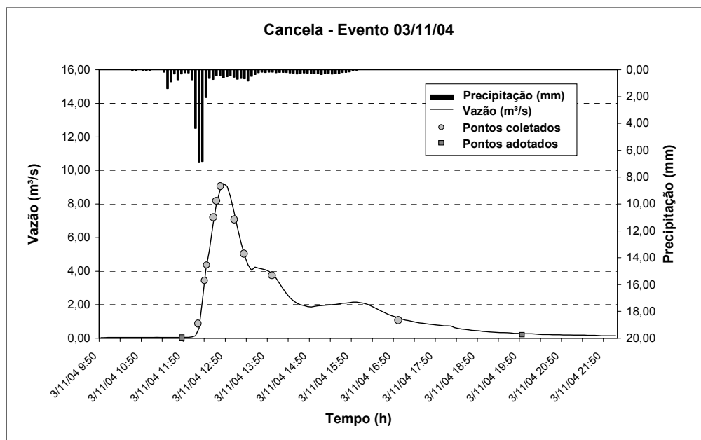
FIGURA 80 – Hidrograma do Evento 03/11/04 – Bacia Hidrográfica Cancela
