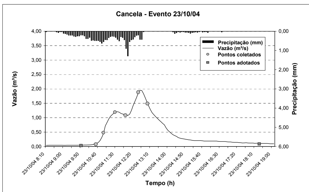
FIGURA 79 – Hidrograma do Evento 23/10/04 – Bacia Hidrográfica Cancela
