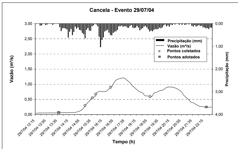
FIGURA 72 – Hidrograma do Evento 29/07/04 – Bacia Hidrográfica Cancela
