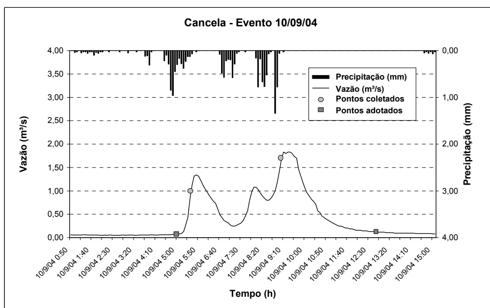
FIGURA 75 – Hidrograma do Evento 10/09/04 – Bacia Hidrográfica Cancela
