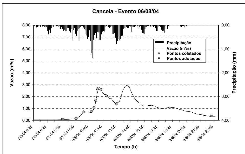
FIGURA 73 – Hidrograma do Evento 06/08/04 – Bacia Hidrográfica Cancela
