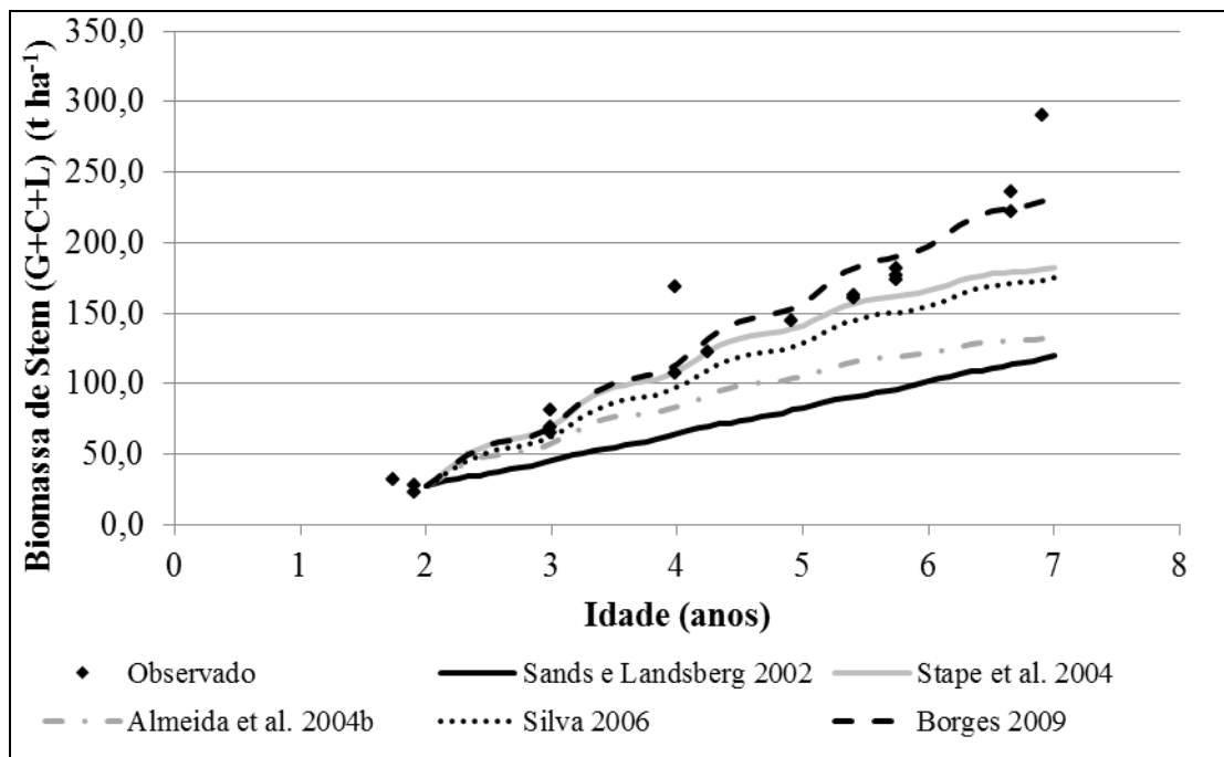
Figura 22 - Biomassa de stem observada e estimada pelo modelo 3-PG, através da parametrização de outros autores.
