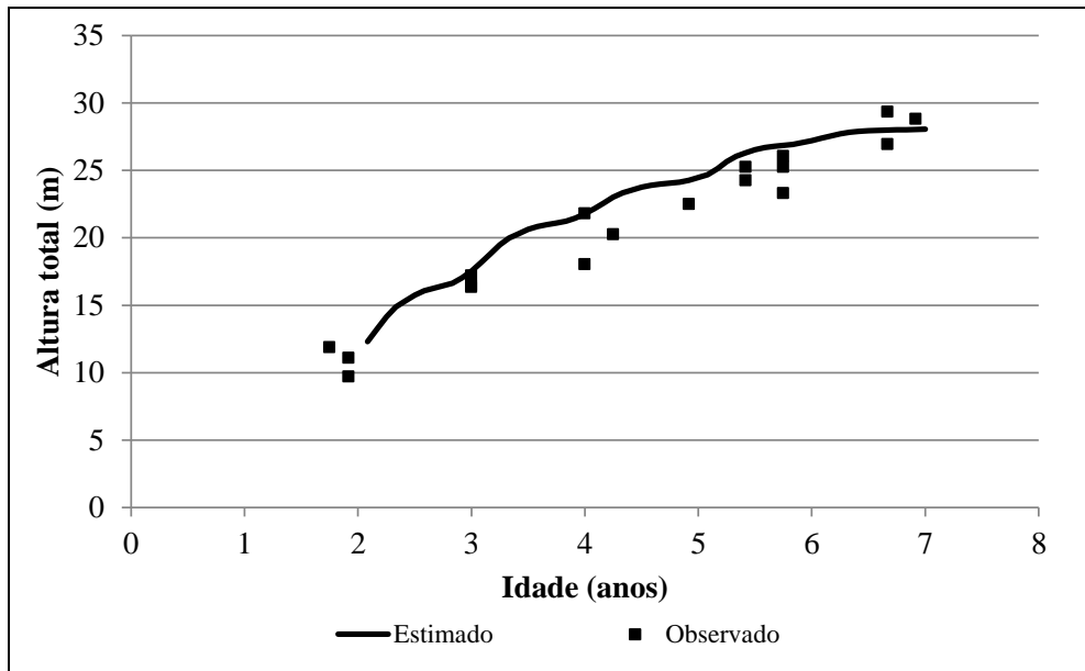
Figura 16 - Valores observados e estimados pelo modelo 3-PG da altura total (m) de E. saligna .
