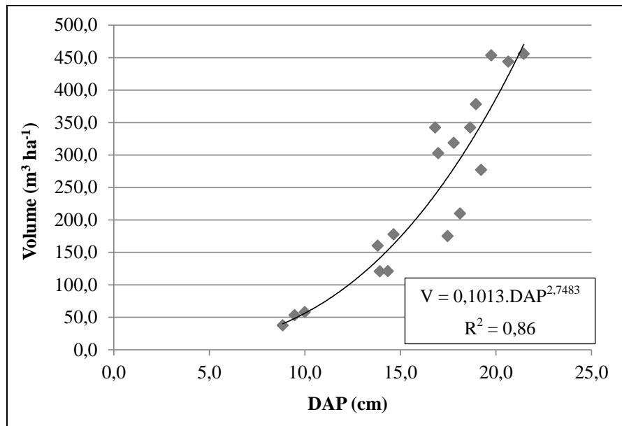
Figura 12 - Equação alométrica ajustada entre o volume de madeira sem casca ( m^3 ha^{-1} ) e o DAP (cm).
