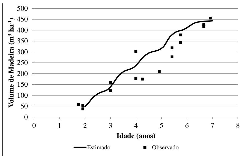
Figura 17 - Valores observados e estimados através do modelo 3-PG para volume de madeira ( \text{m}^3 \text{ha}^{-1} ) de E. saligna .
