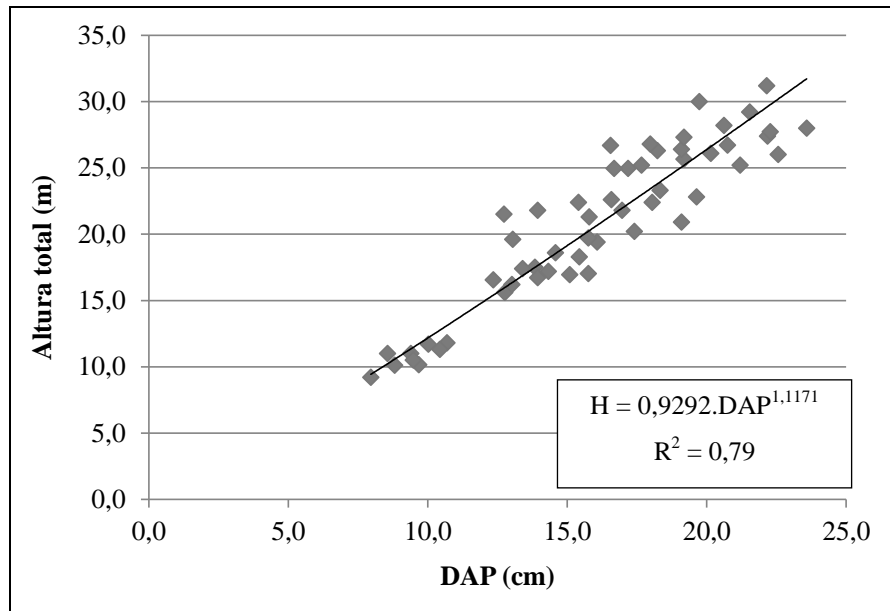
Figura 11 - Equação alométrica ajustada entre a altura total (m) e o DAP (cm).
