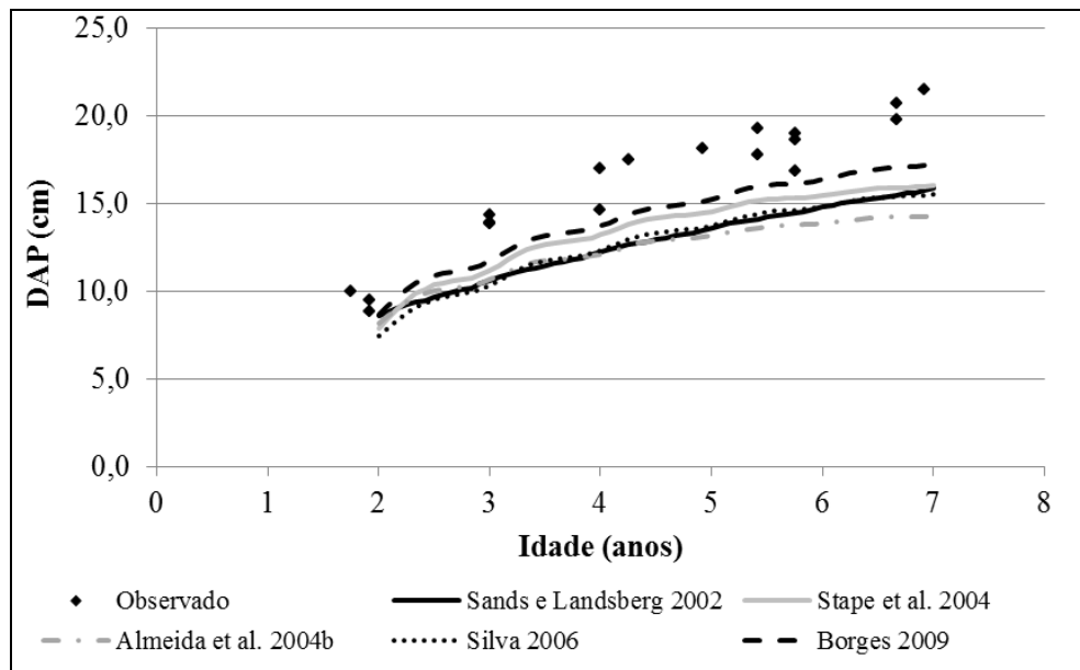
Figura 19 – Diâmetro à altura do peito (DAP) observado e estimado pelo modelo 3-PG, através da parametrização de outros autores.
