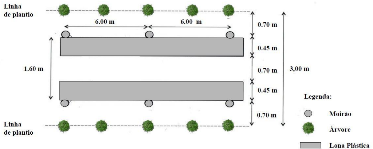
Figura 4 – Esquema ilustrativo do sistema de exclusão da precipitação interna (CE) na área experimental em Telêmaco Borba, PR
