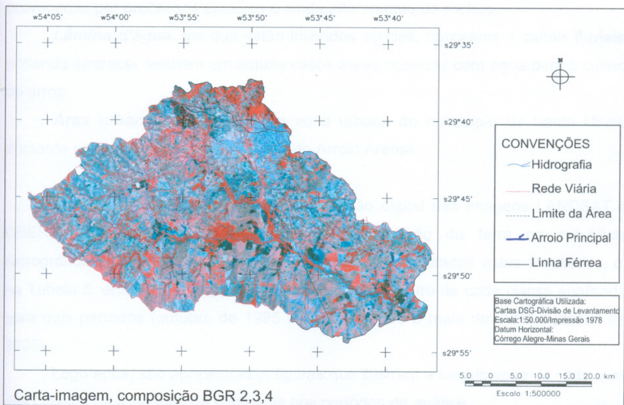
Figura 11 – Carta-imagem, composição BGR 2,3,4 da sub-bacia do Arroio Arenal em janeiro de 2005.
