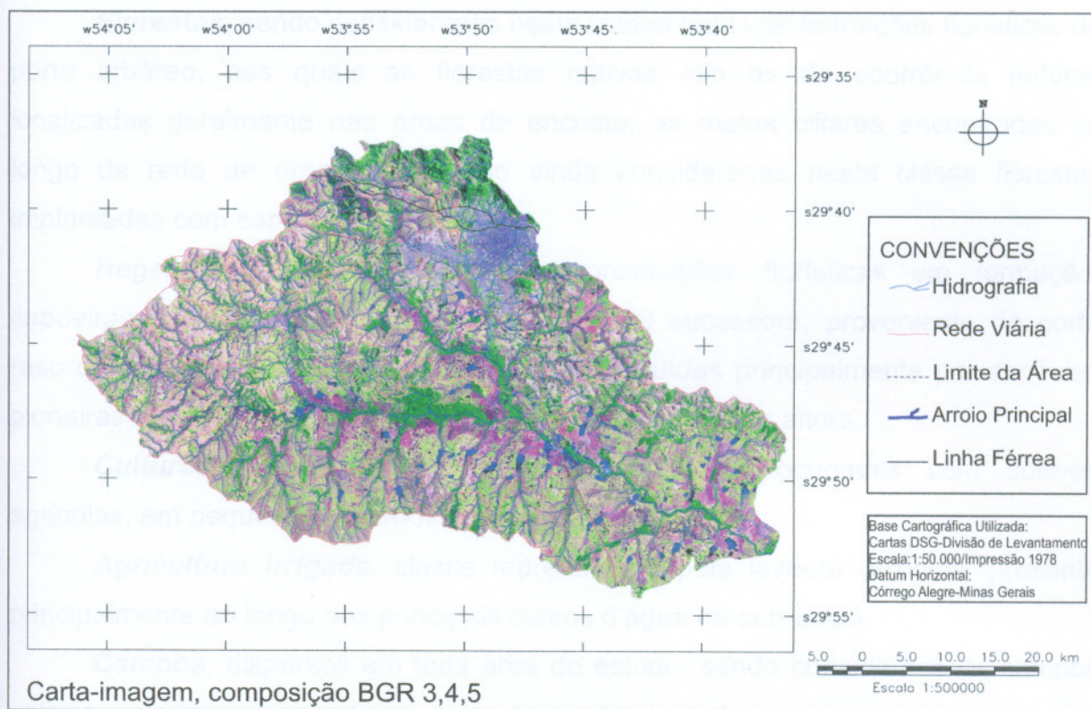
Figura 10 – Carta-imagem, composição BGR 3,4,5 da sub-bacia do Arroio Arenal em outubro de 1995.
