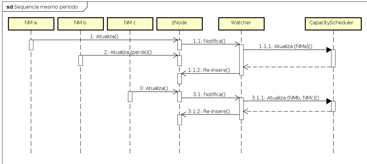
Figura 3.3 – Diagrama de seqüência de uma notificação perdida quando a próxima notificação ocorre na mesma fase de coleta.
