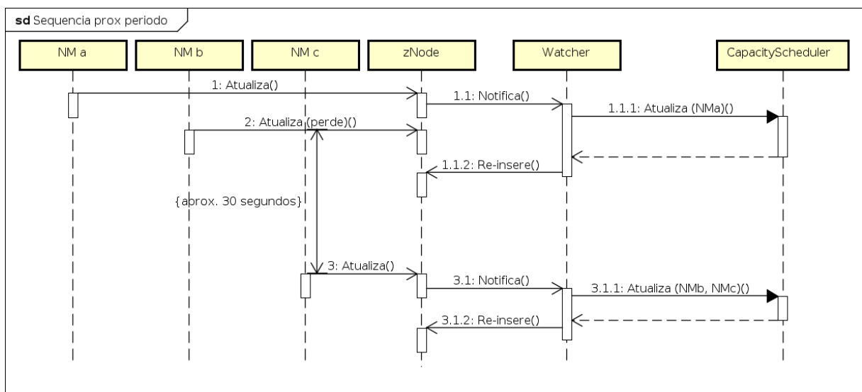
Figura 3.4 – Diagrama de seqüência de uma notificação perdida quando a próxima notificação ocorre na próxima fase de coleta.
