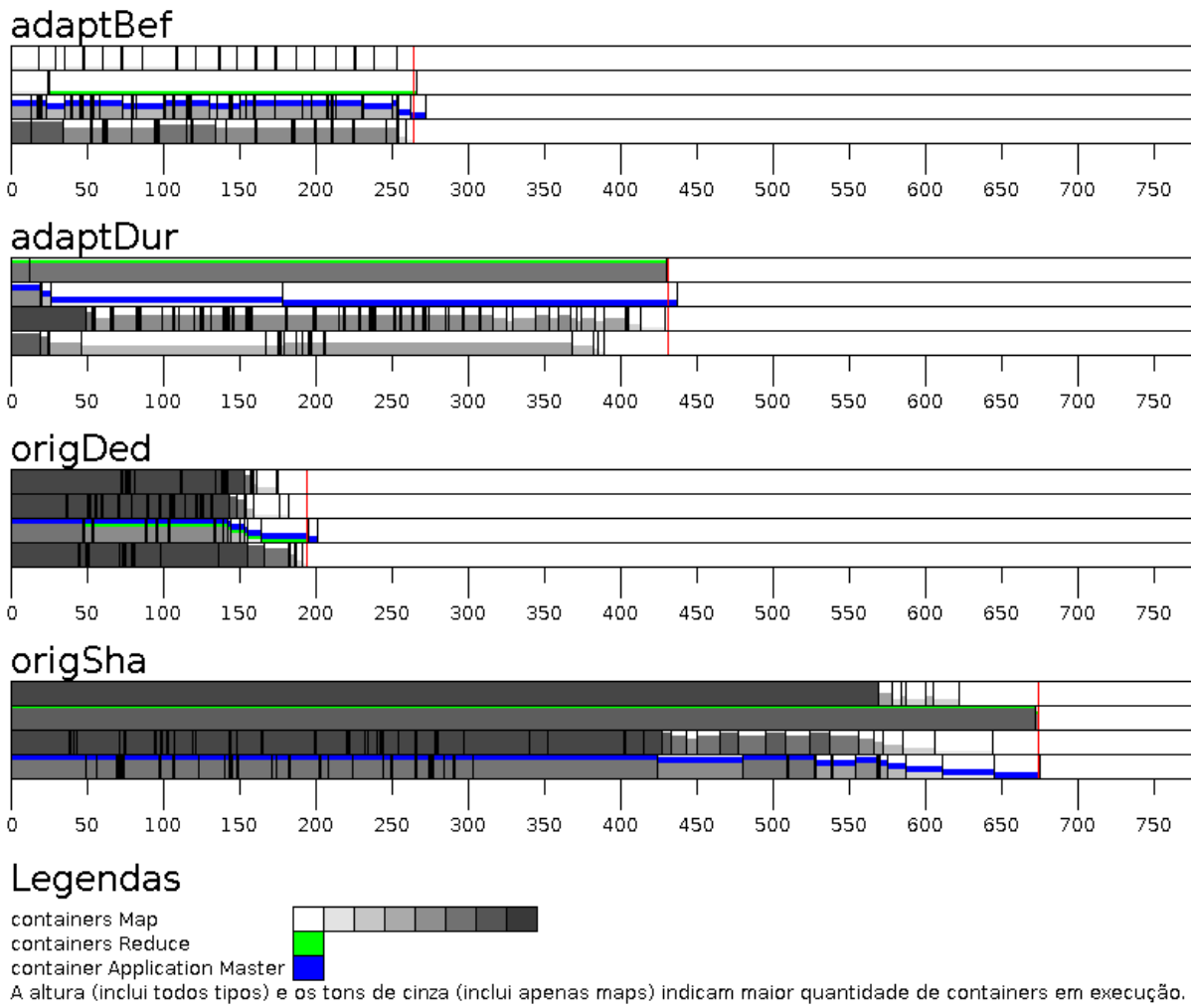
Figura 4.5 – Diagrama de Gantt para os experimentos concorrentes com TestDFSIO
