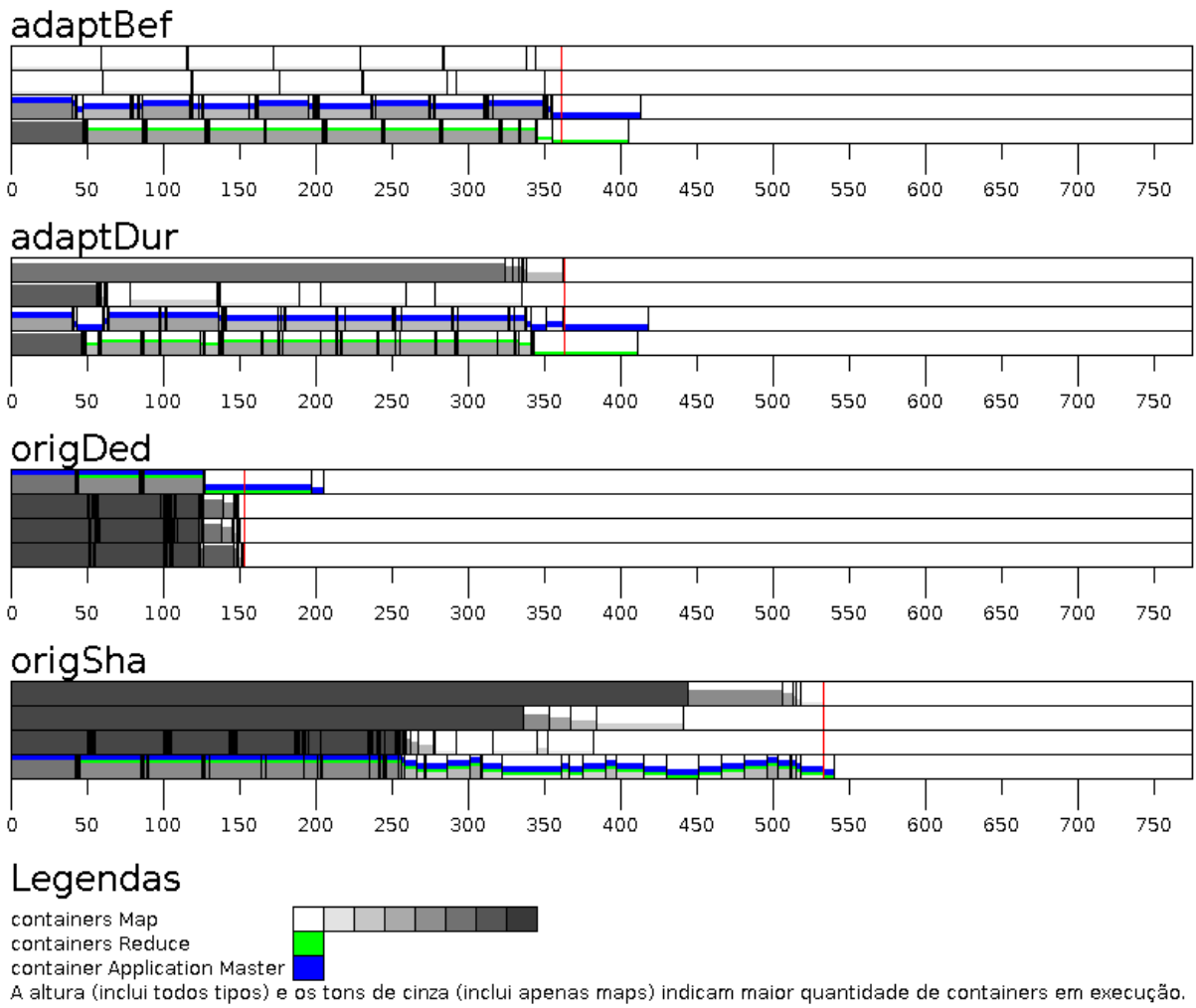
Figura 4.6 – Diagrama de Gantt para os experimentos concorrentes com WordCount
