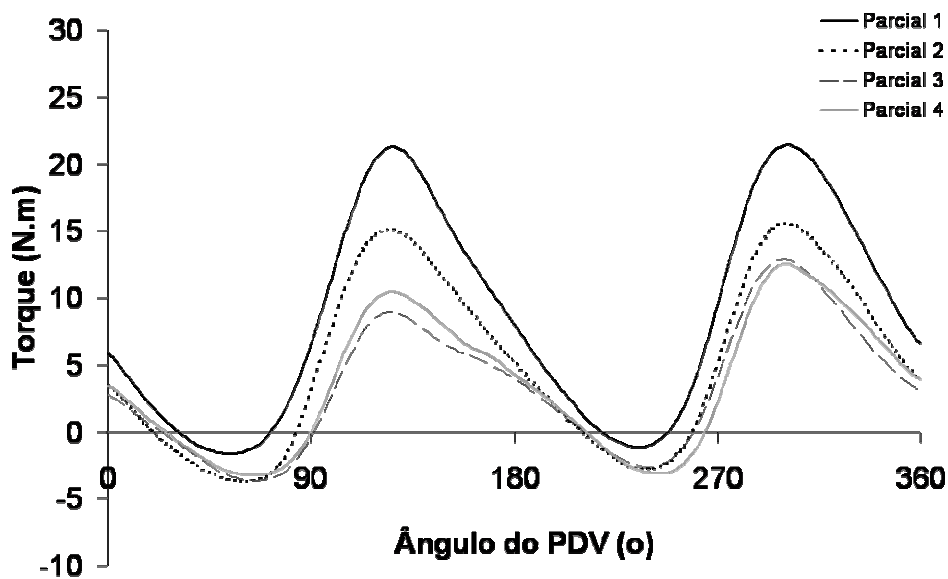
Figura 4.8: Padrão de torque para o ciclista 5.
