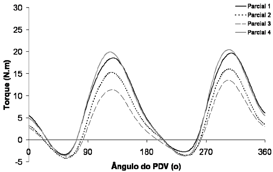
Figura 4.6: Padrão de torque para o ciclista 3.
