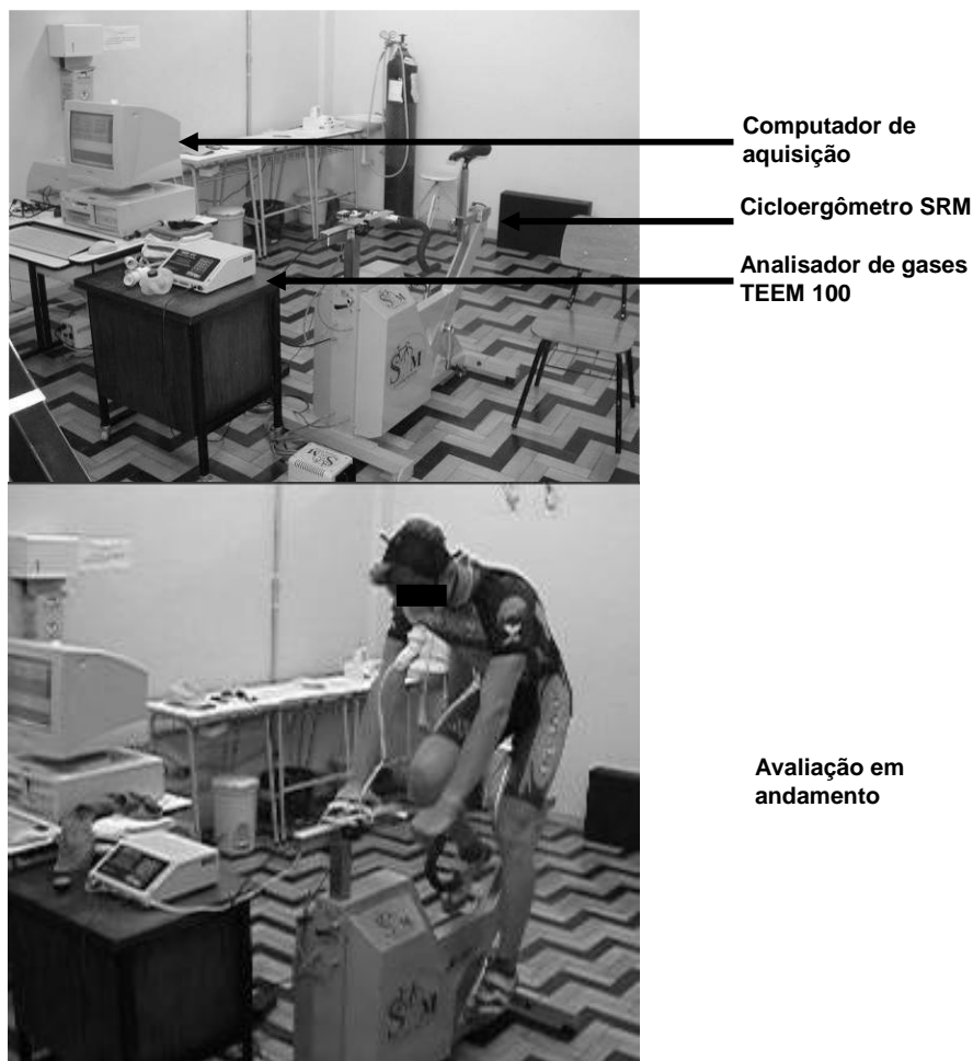
Figura 3.2: Ambiente de coleta dos dados
