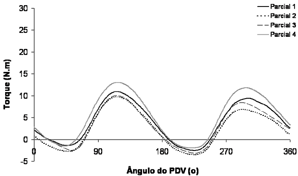
Figura 4.4: Padrão de torque para o ciclista 1.
