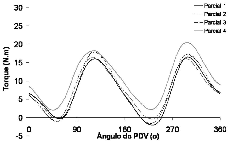
Figura 4.7: Padrão de torque para o ciclista 4.
