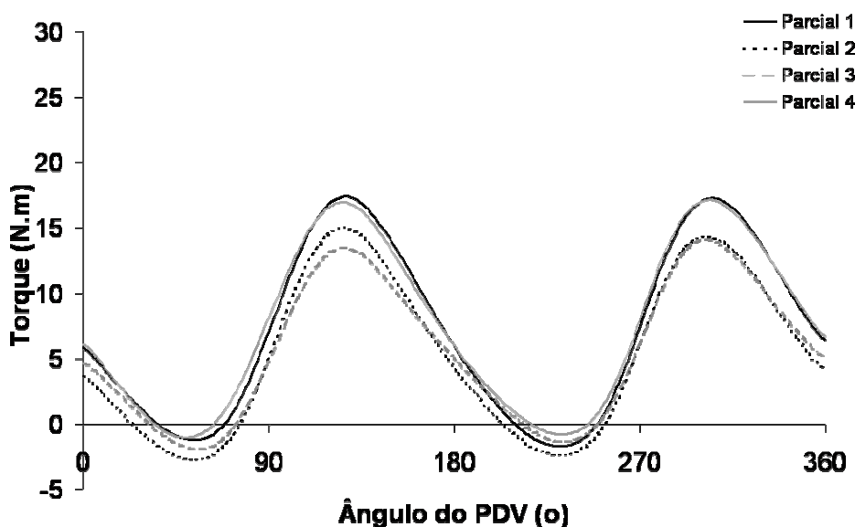
Figura 4.2: Torque produzido pelo grupo a cada 5 minutos
