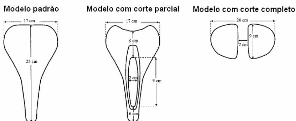
Figura 2.2: Desenhos de selins, adaptado de Bressel & Larson (2003).
