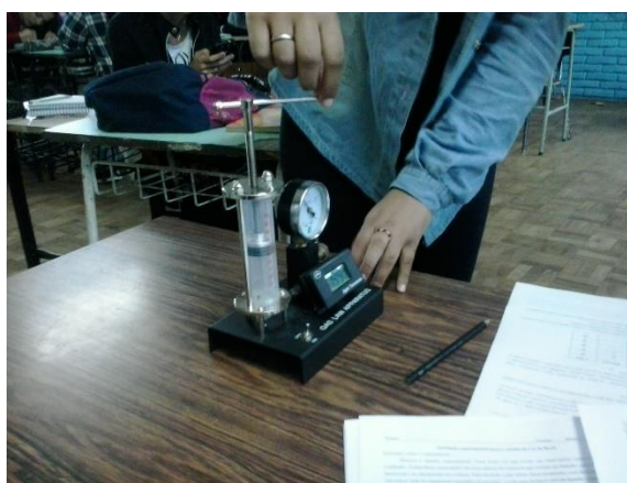
Figura 24 – Realização do experimento sobre Robert Boyle
