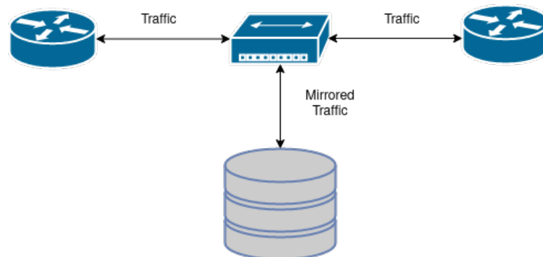
Figura 2.9 – Monitoramento passivo
