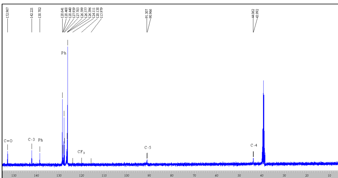
Figura 59: Espectro de RMN ^1\text{H} a 200,13 MHz e ^{13}\text{C}\{\text{H}\} a 100,61 MHz do composto (6j), em \text{DMSO-}d_6 .
