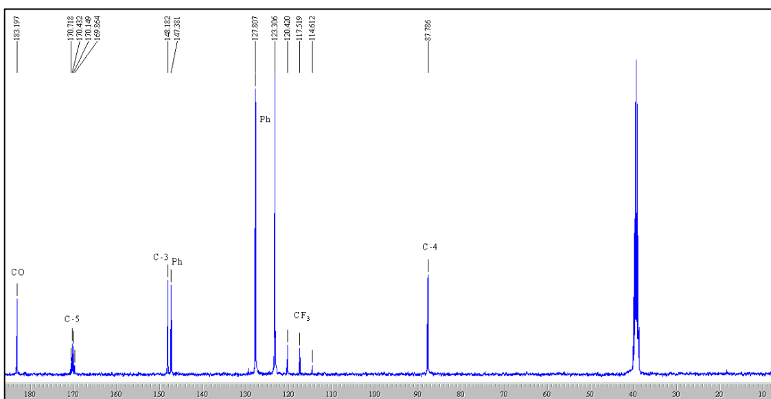
Figura 44: Espectro de RMN 1 H a 200,13 MHz e 13 C{H} a 100,61 MHz do composto (3i), em DMSO- d 6 .
