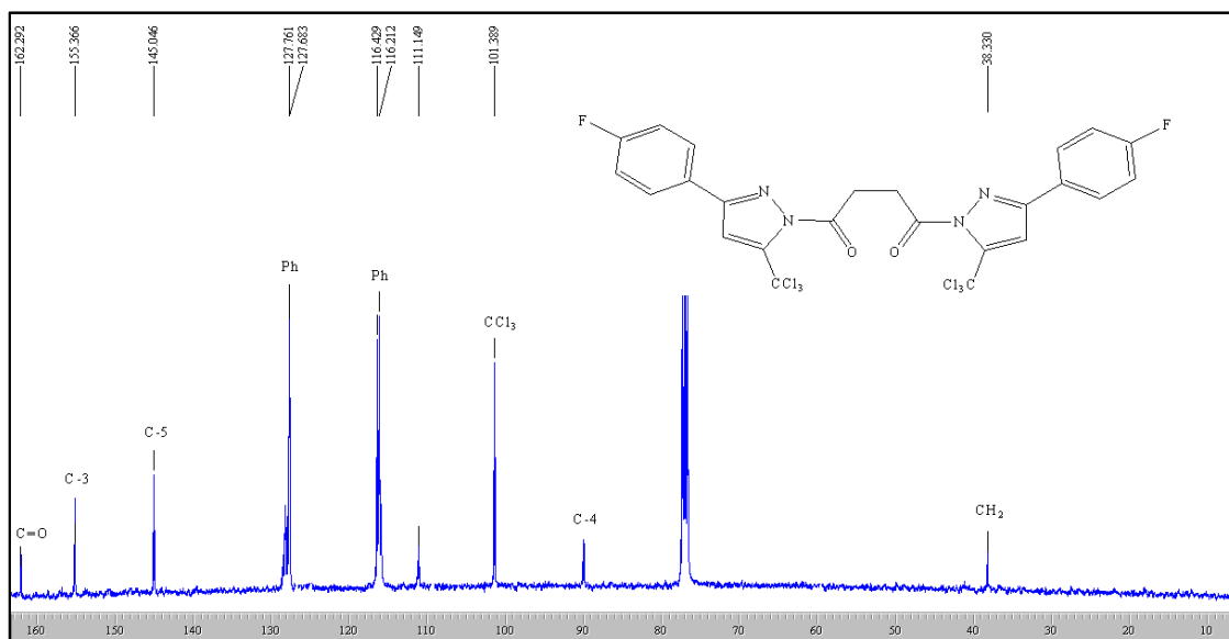
Figura 86: Espectro de RMN ^1\text{H} a 200,13 MHz e ^{13}\text{C}\{\text{H}\} a 100,61 MHz do composto ( 15f ), em \text{DMSO}-d_6 .
