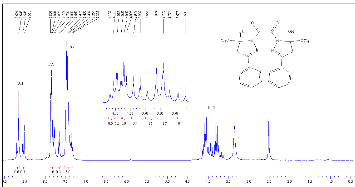
Figura 18: Espectro de RMN ^1\text{H} a 200,13 MHz de Oxalil-1,1'-Bis-3-fenil-5-triclorometil-5-hidróxi-4,5-diidro-1 H -pirazol ( 8c ), em \text{DMSO-}d_6 .
