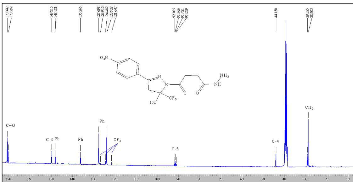
Figura 78: Espectro de RMN ^1\text{H} a 200,13 MHz e ^{13}\text{C}\{\text{H}\} a 100,61 MHz do composto (12i), em \text{DMSO-}d_6 .
