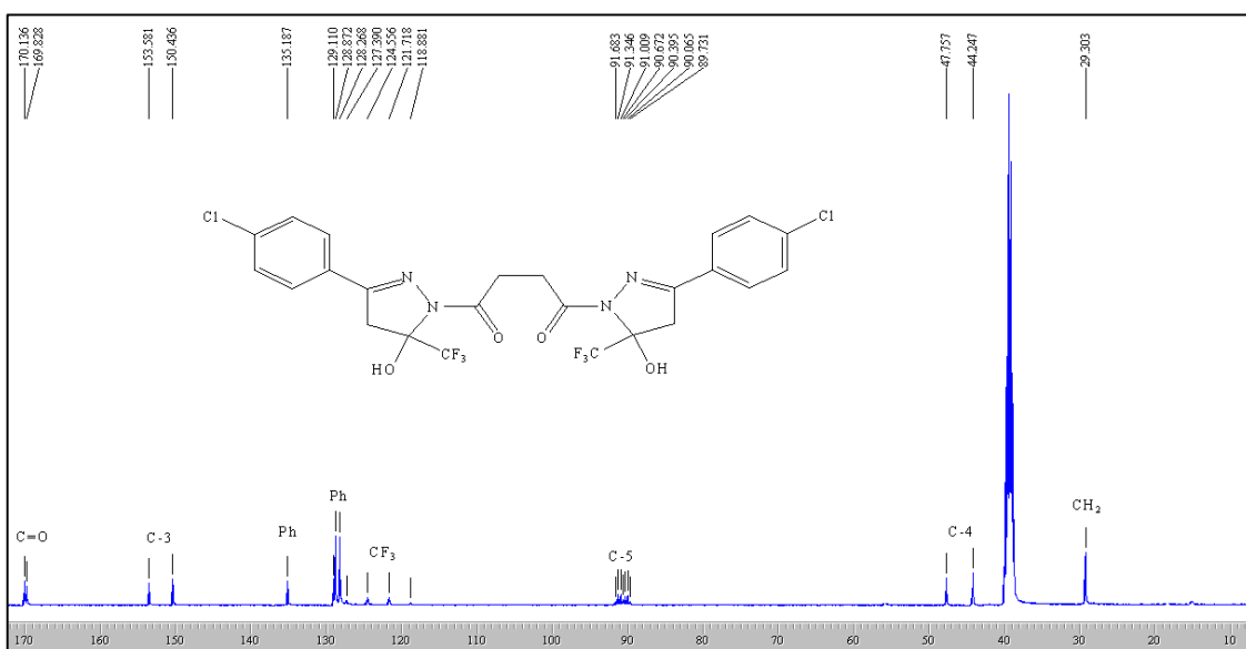
Figura 73: Espectro de RMN 1 H a 200,13 MHz e 13 C{H} a 100,61 MHz do composto (10g), em DMSO- d 6 .
