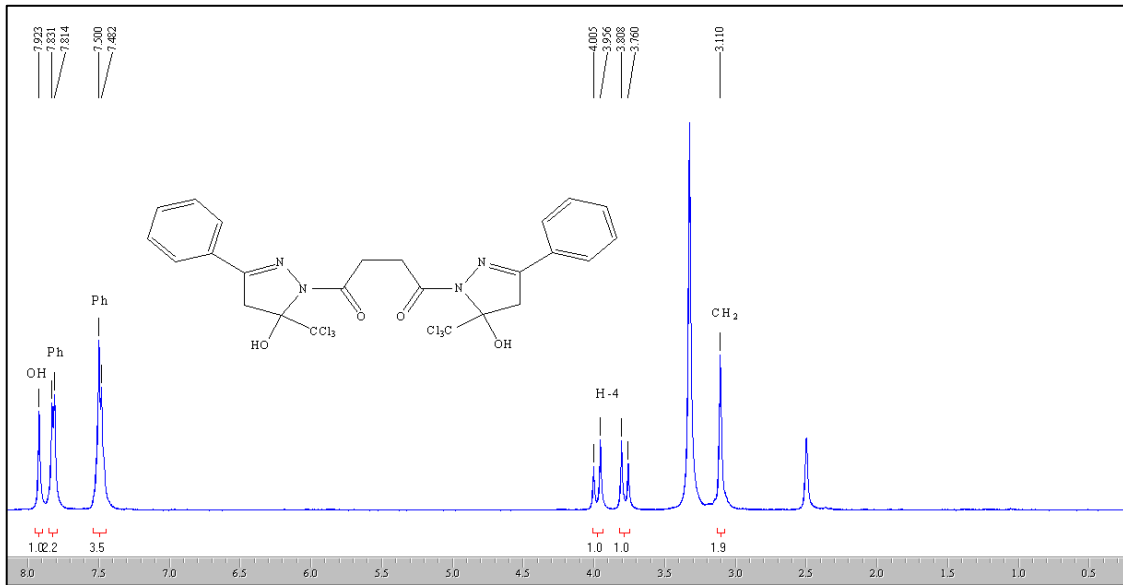
Figura 32: Espectro de RMN ^1\text{H} a 200,13 MHz de Succinil-1,1'-Bis-5-triclorometil-3-fenil-5-hidroxi-4,5-diidro-1H-pirazol ( 14c ), em \text{DMSO}-d_6 .
