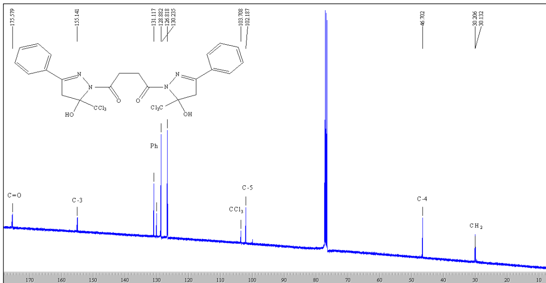
Figura 33: Espectro de RMN ^{13}\text{C}\{\text{H}\} a 100,61 MHz de Succinil-1,1'-Bis-5-triclorometil-3-fenil-5-hidroxi-4,5-diidro-1H-pirazol ( 14c ), em \text{CDCl}_3-d_1 .
