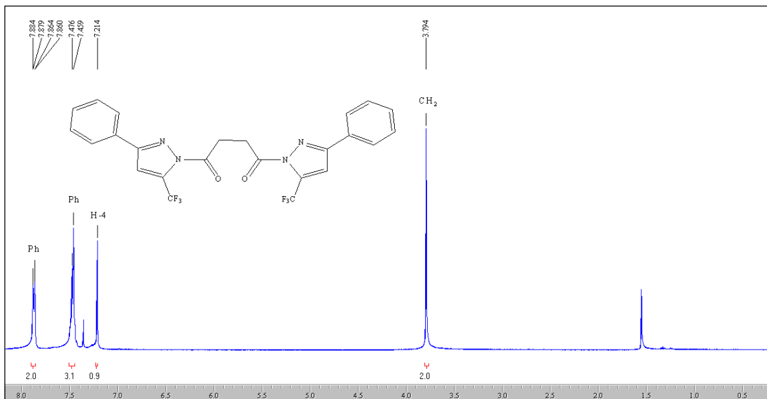
Figura 25: Espectro de RMN ^1\text{H} a 200,13 MHz de Succinil-1,1'-Bis-3-fenil-5-trifluorometil-1 H -pirazol ( 11c ), em \text{CDCl}_3-d_1
