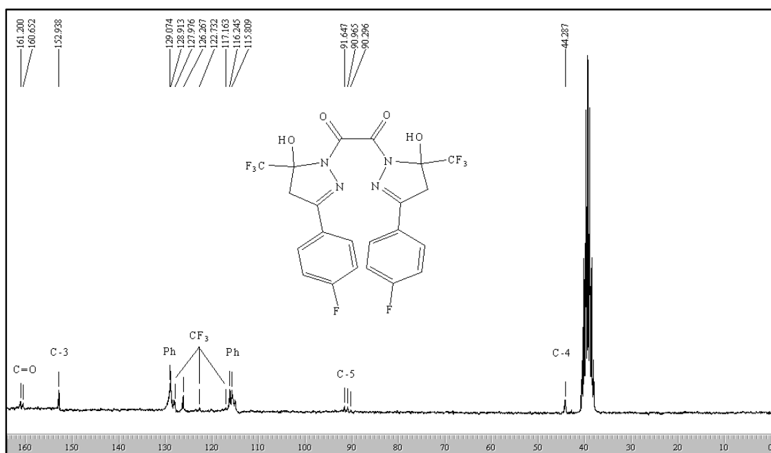
Figura 56: Espectro de RMN ^1\text{H} a 200,13 MHz e ^{13}\text{C}\{\text{H}\} a 100,61 MHz do composto (6f), em \text{DMSO}-d_6 .
