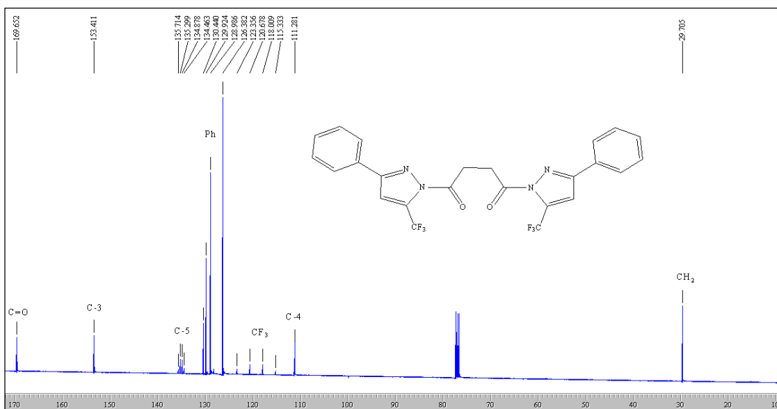
Figura 26: Espectro de RMN ^{13}\text{C} \{^1\text{H}\} a 100,61 MHz de Succinil-1,1'-Bis-3-fenil-5-trifluorometil-1 H -pirazol ( 11c ), em \text{CDCl}_3-d_1
