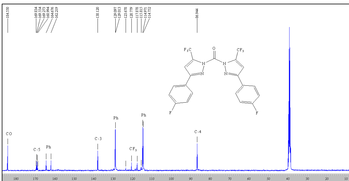
Figura 43: Espectro de RMN ^1\text{H} a 200,13 MHz e ^{13}\text{C}\{\text{H}\} a 100,61 MHz do composto (3f), em \text{DMSO-}d_6 .
