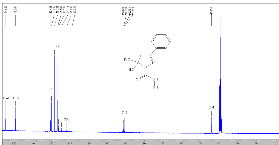
Figura 92: Espectro de RMN ^1\text{H} a 200,13 MHz e ^{13}\text{C}\{\text{H}\} a 100,61 MHz do composto ( 18c ), em \text{DMSO-}d_6 .
