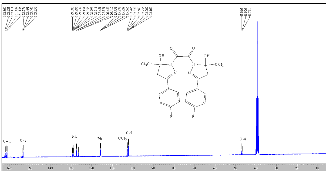
Figura 64: Espectro de RMN 1 H a 200,13 MHz e 13 C{H} a 100,61 MHz do composto (8f), em DMSO-d 6 .
