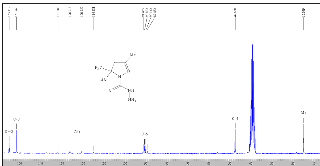
Figura 91: Espectro de RMN ^1\text{H} a 200,13 MHz e ^{13}\text{C}\{\text{H}\} a 100,61 MHz do composto (18b), em \text{DMSO-}d_6 .
