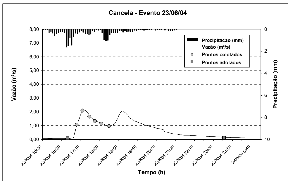
FIGURA 70 – Hidrograma do Evento 23/06/04 – Bacia Hidrográfica Cancela
