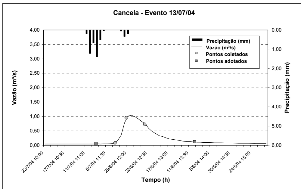
FIGURA 71 – Hidrograma do Evento 13/07/04 – Bacia Hidrográfica Cancela
