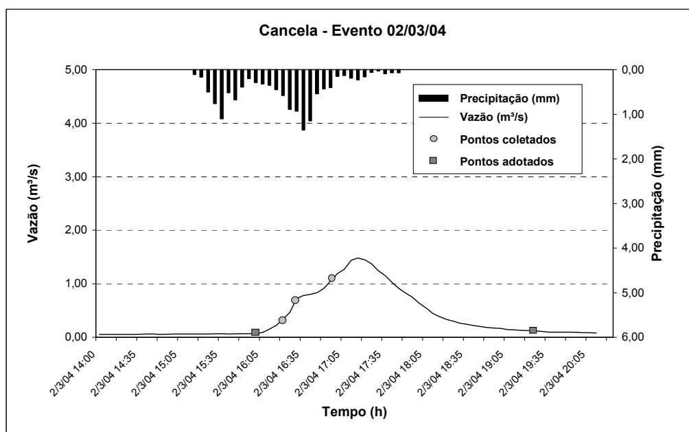
FIGURA 65 – Hidrograma do Evento 02/03/04 – Bacia Hidrográfica Cancela
