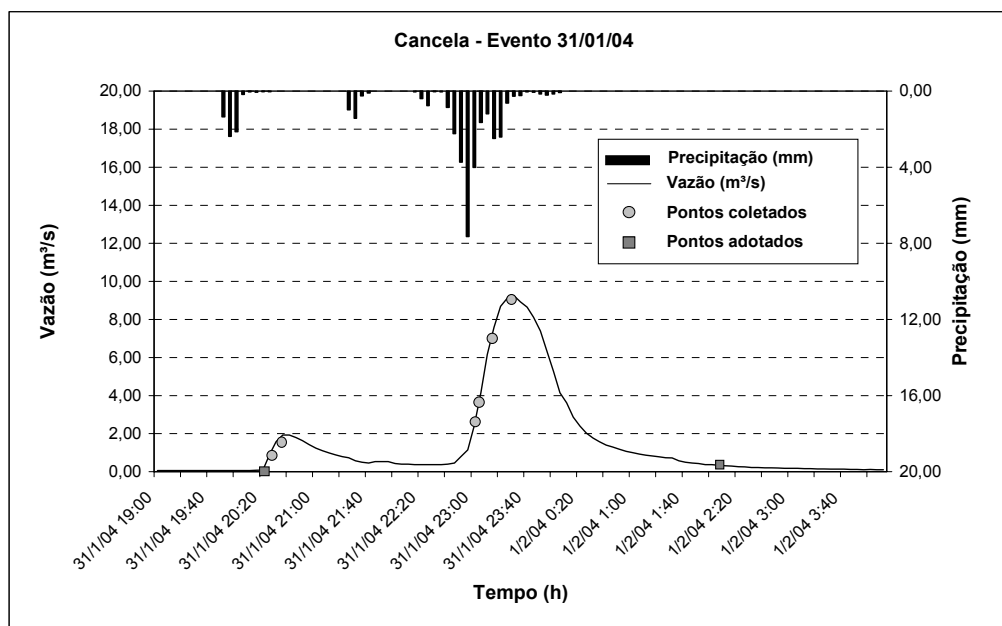
FIGURA 64 – Hidrograma do Evento 31/01/02 – Bacia Hidrográfica Cancela
