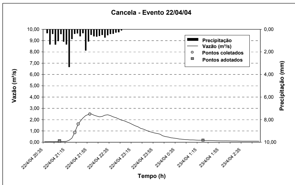
FIGURA 68– Hidrograma do Evento 22/04/04 – Bacia Hidrográfica Cancela
