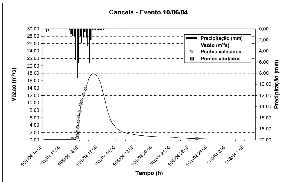
FIGURA 69 – Hidrograma do Evento 10/06/04 – Bacia Hidrográfica Cancela
