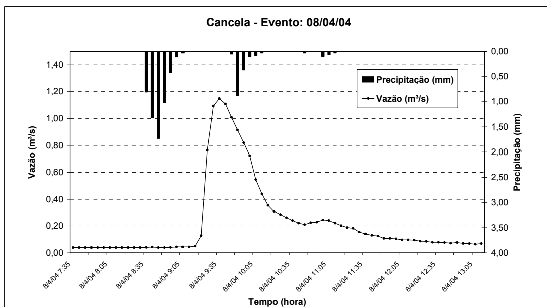
FIGURA 67 – Hidrograma do Evento 08/04/04 – Bacia Hidrográfica Cancela
