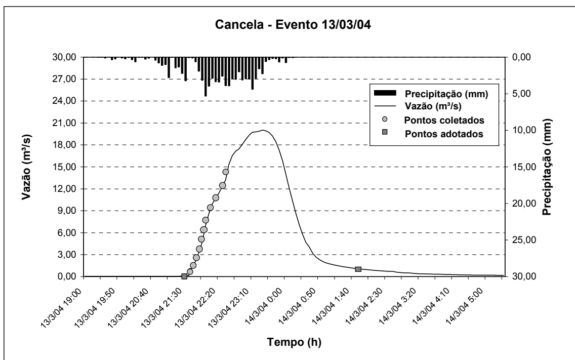
FIGURA 66 – Hidrograma do Evento 13/03/04 – Bacia Hidrográfica Cancela
