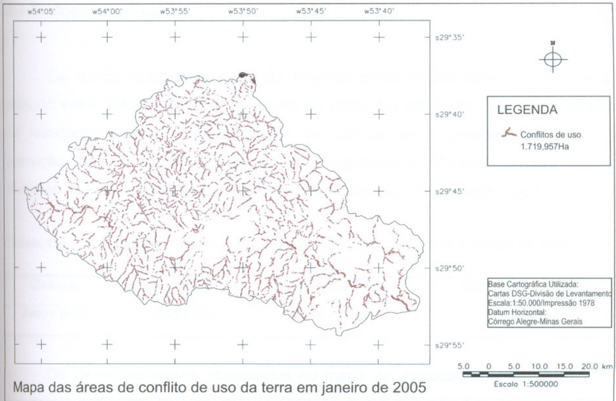
Figura 24 – Áreas de conflito de uso da terra na sub-bacia do Arroio Arenal em janeiro de 2005.
