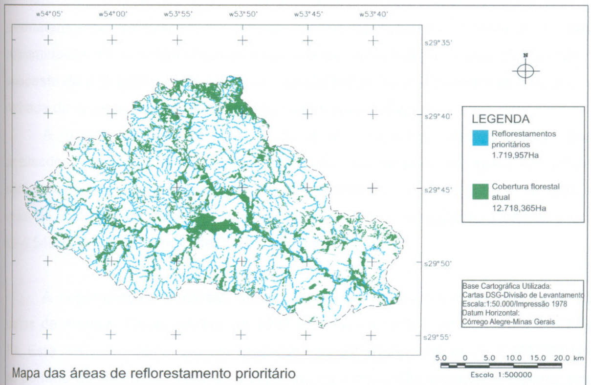
Figura 25 – Áreas de reflorestamento prioritário na sub-bacia do Arroio Arenal em janeiro de 2005.
